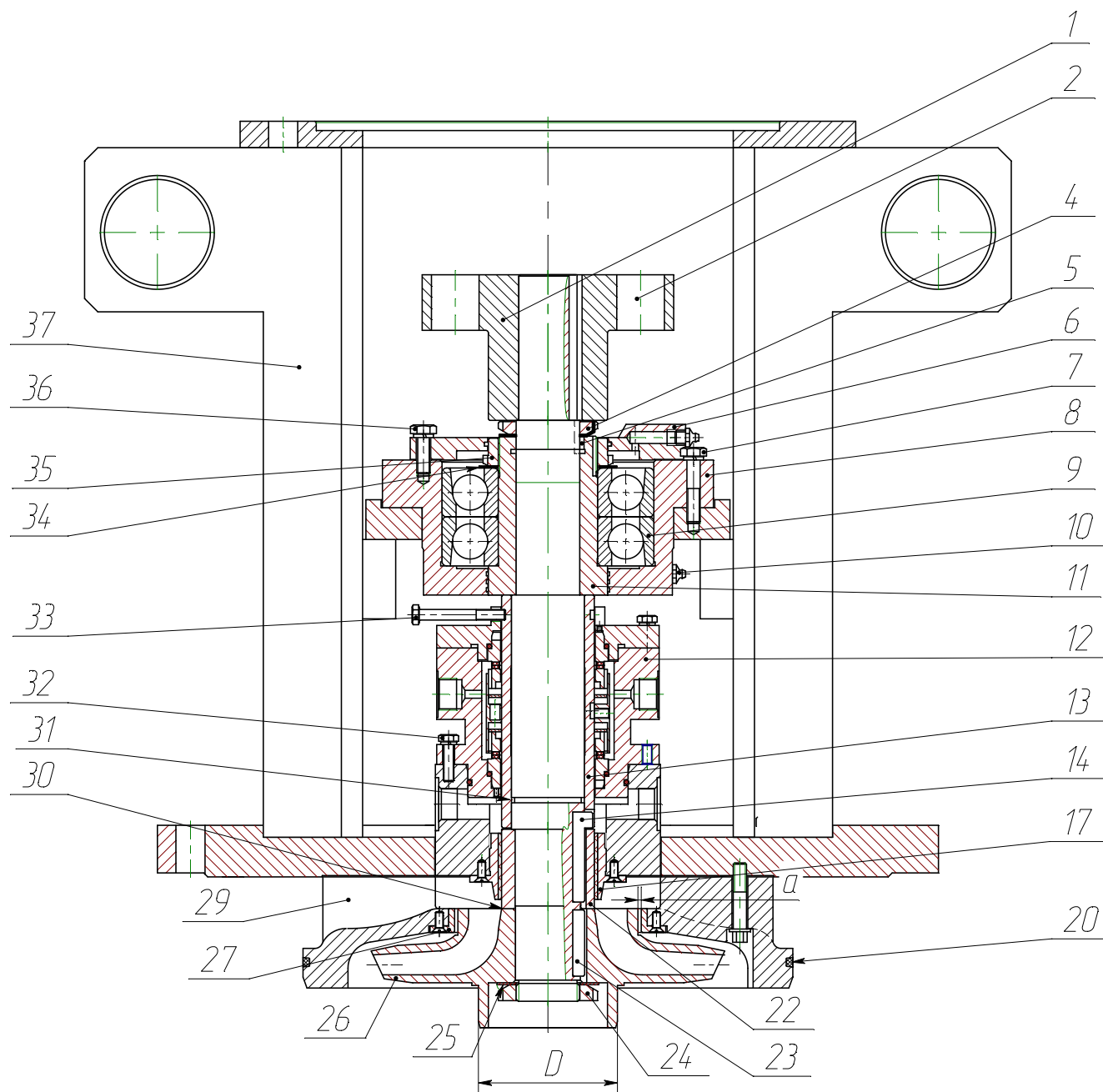
Рисунок 2-1- Быстроходная часть насосов (агрегатов) 1КсВ125-71-..., 1КсВ315-80-...
