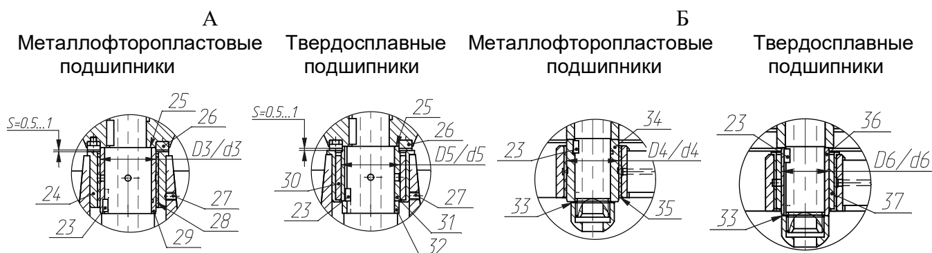
Рисунок 1-2 – Тихоходная часть насосов (агрегатов) типа 1КсВ
